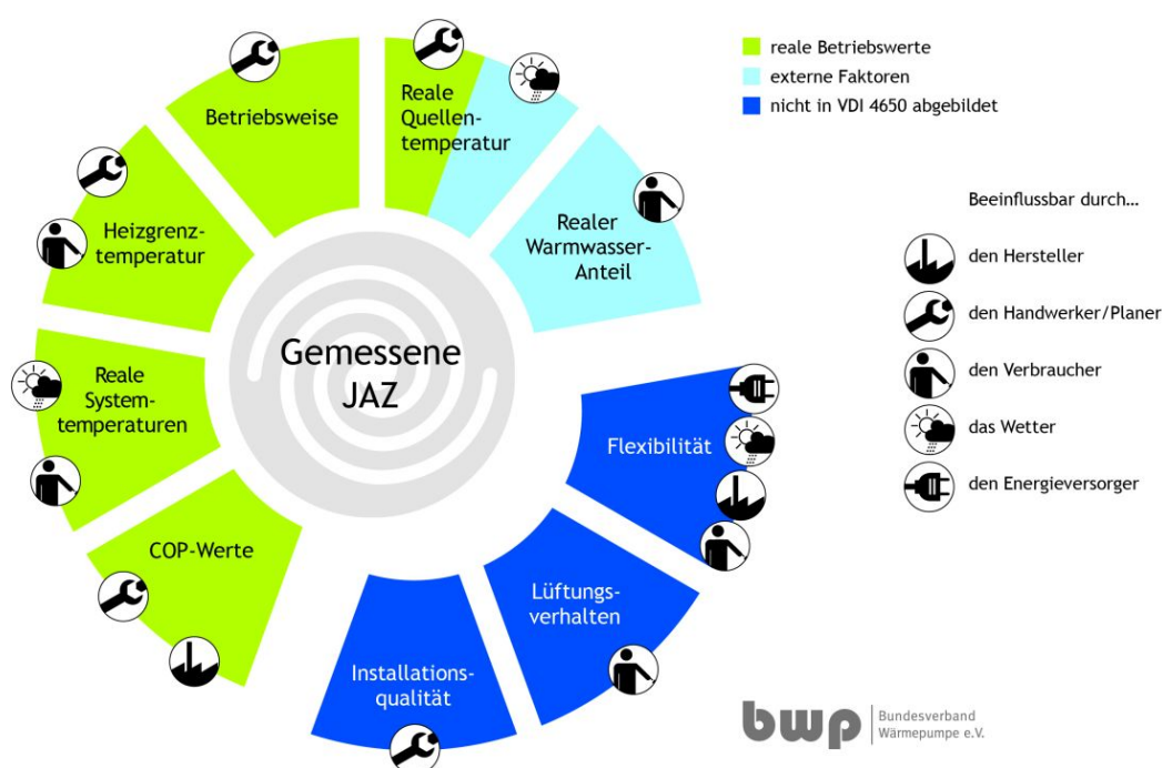
Einflussgrößen auf die Effizienz von Wärmepumpen
